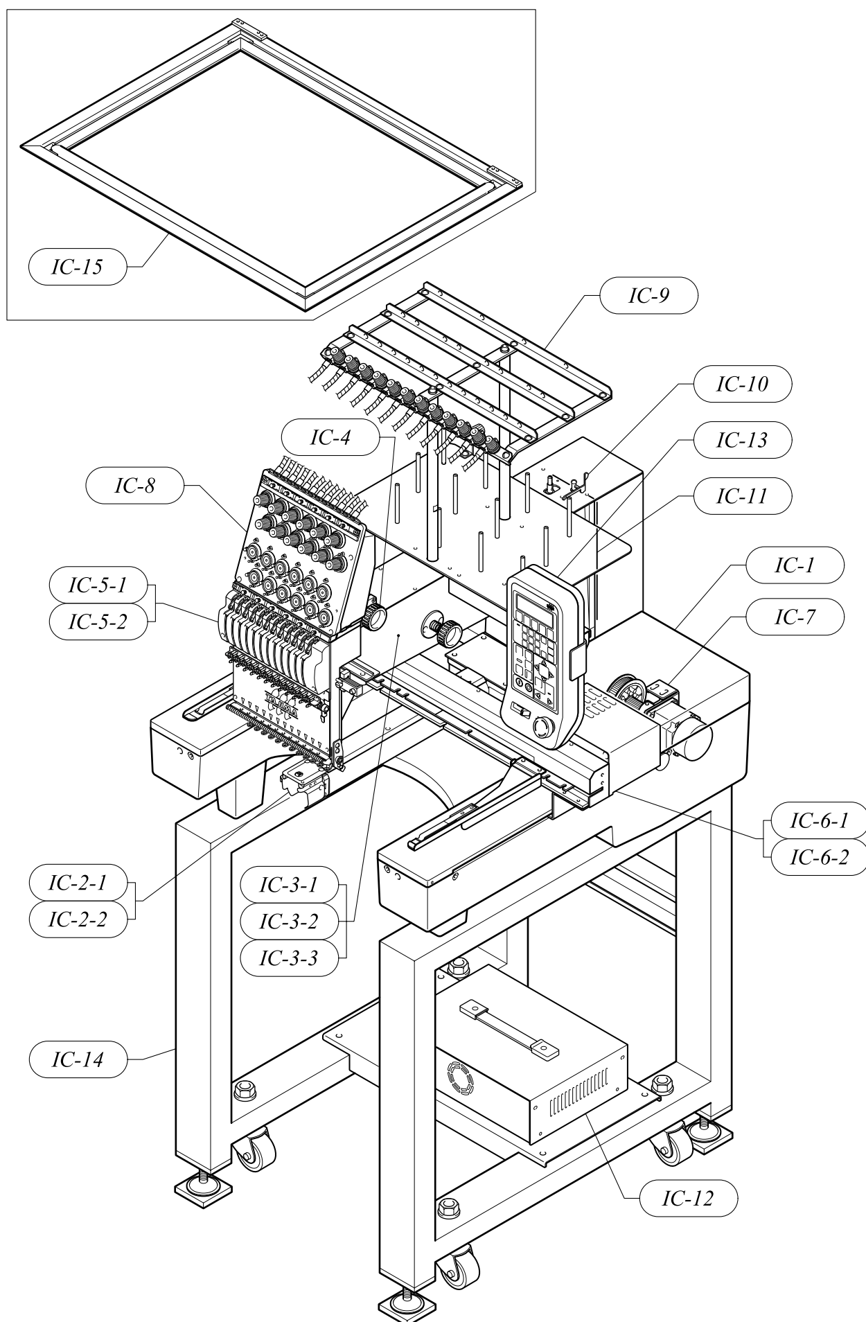
全体図 GENERAL VIEW
